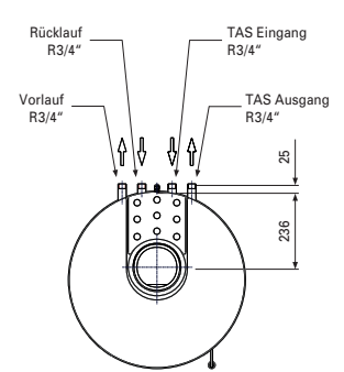
Draufsicht
