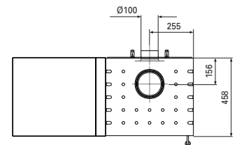
Draufsicht ⓪
