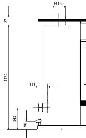
Seitenansicht
