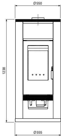
Frontansicht
