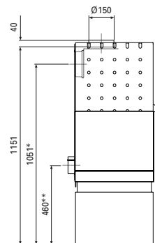
Seitenansicht ⓪
