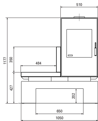
Frontansicht ⓪
